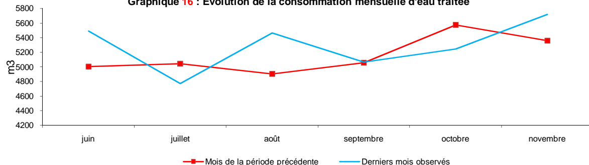
Graphique 16 : Evolution de la consommation mensuelle d'eau traitée
