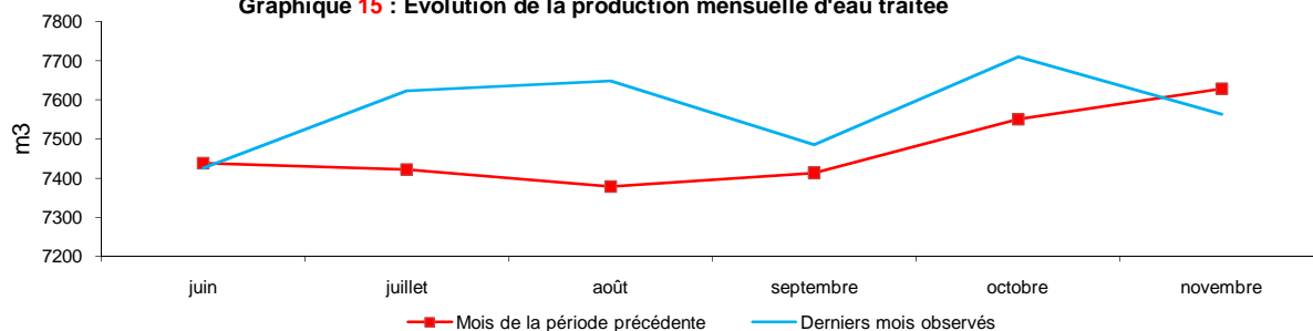
Graphique 15 : Evolution de la production mensuelle d'eau traitée
